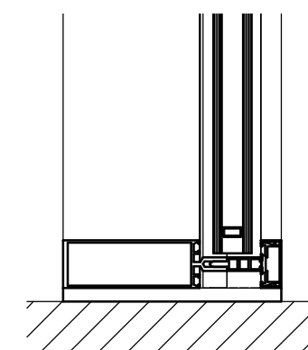
8 Detail 6 1 : 5
